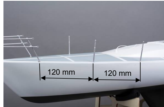
Abb. Relingstützen einbauen
